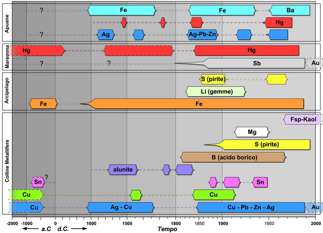
Figura 2 - Diagramma che mostra l'utilizzo delle risorse minerarie, divise per distretti minerari, nelle diverse epoche storiche e preistoriche della Toscana. I colori e i simboli per i vari distretti sono gli stessi utilizzati in Figura 1. Altre abbreviazioni
