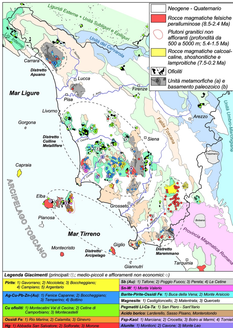
Figura 1- Carta geologica schematica della Toscana con indicati i principali distretti minerari del passato e le varie tipologie di giacimenti minerari presenti.
